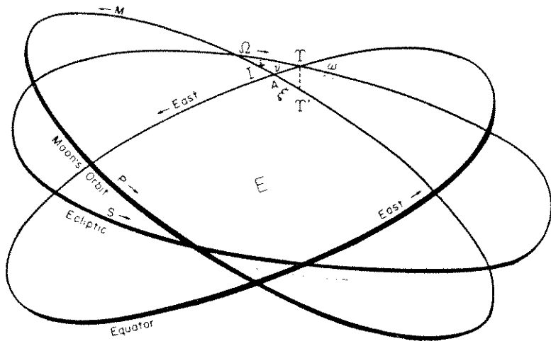
FIG. 1—Orbital parameters.
